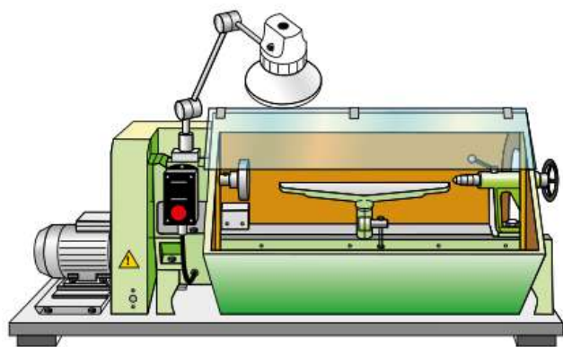
Рис. 3.3. Токарный станок для обработки древесины
