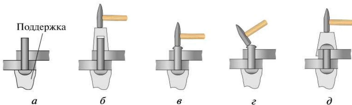
Рис. 5.47. Соединение деталей заклёпками с полукруглой головкой:
