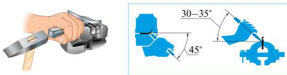
Рис. 5.20. Рубка в тисках по уровню губок
