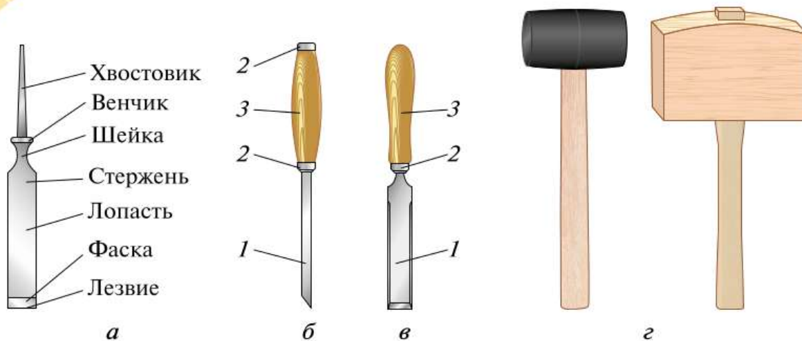
Рис. 4.53. Инструменты для долбления:
