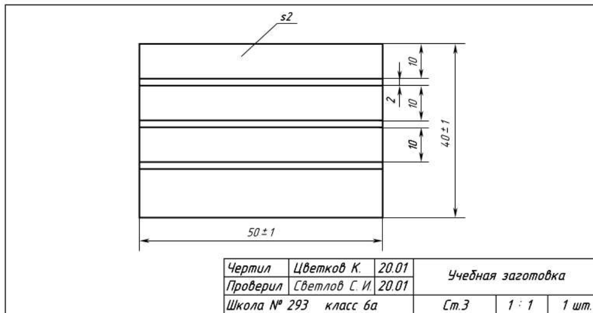
Рис. 5.22. Чертёж учебной заготовки для рубки полос
