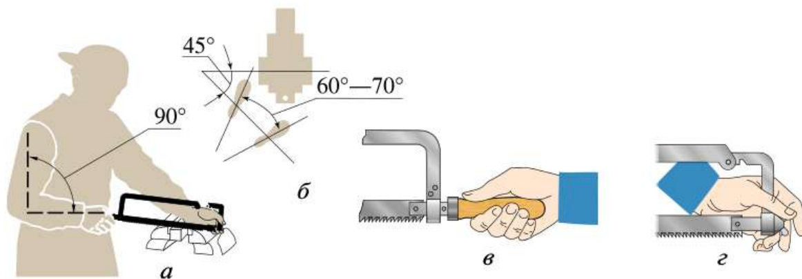
Рис. 5.26. Рабочее положение при резании слесарной ножовкой:
