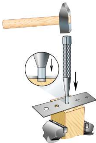
Рис. 5.48. Пробивание отверстий бородком
