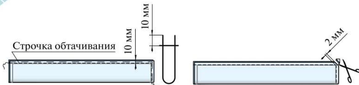
Рис. 6.34. Обработка деталей
