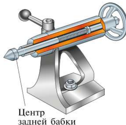
Рис. 5.44. Конусное соединение центра задней бабки
