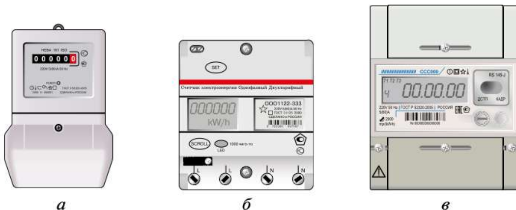
Рис. 11.11. Однофазные счётчики электрической энергии: а — однотарифный; б — двухтарифный; в — многотарифный
