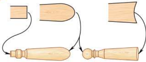
Рис. 4.38. Торцевание концов заготовки
