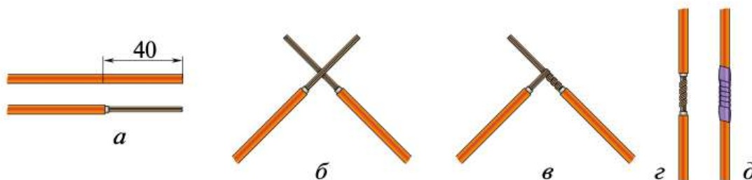
Рис. 11.4. Последовательность сращивания многожильных проводов
