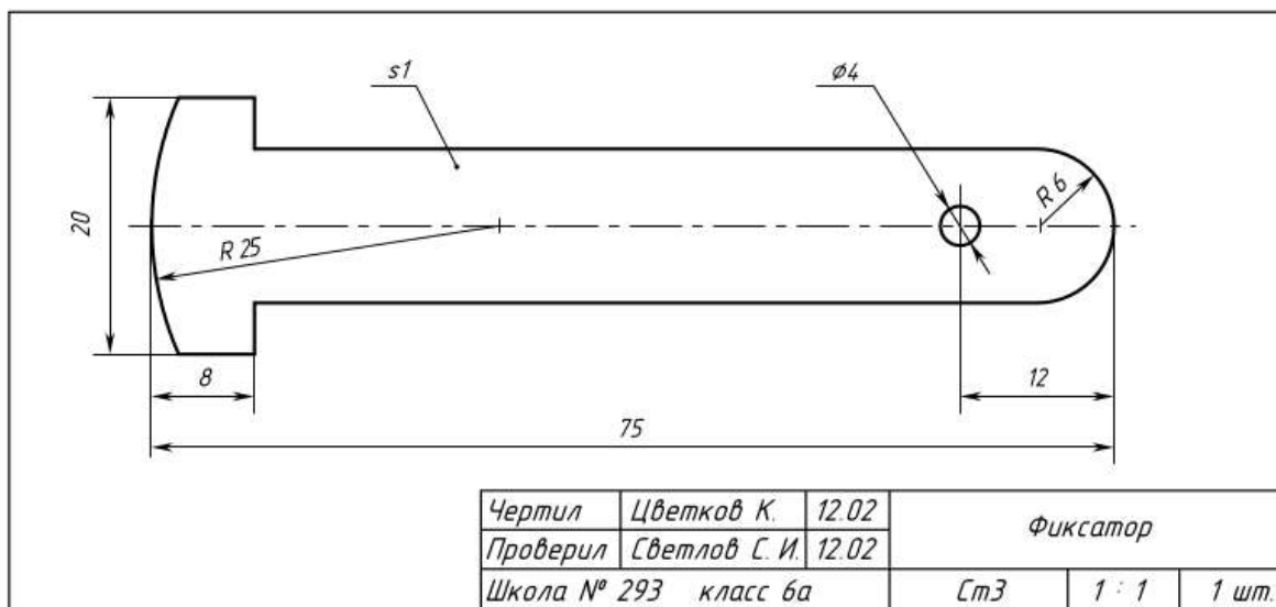
Рис. 5.40. Чертеж фиксатора
