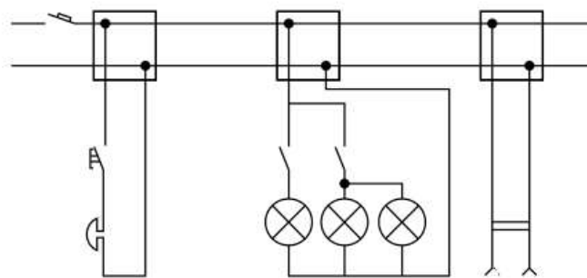
Рис. 11.13. Электрическая схема квартирной электропроводки
