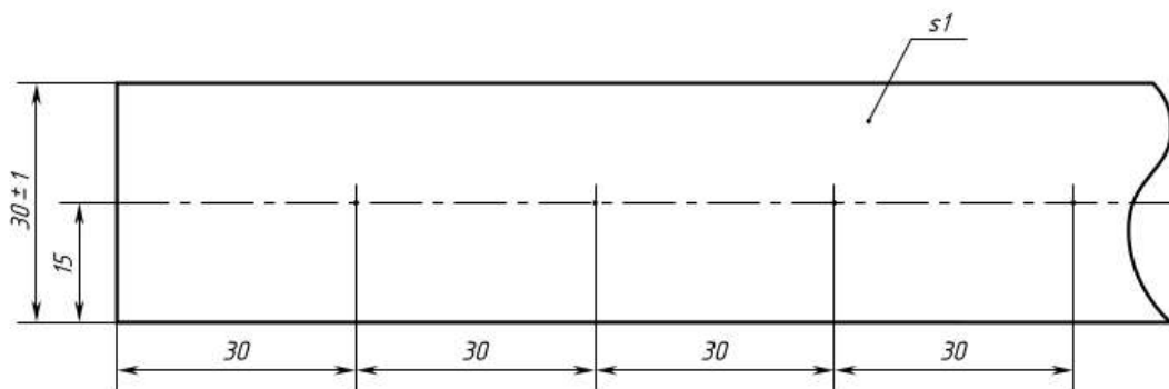
Рис. 5.54. Учебная заготовка для заклёпочного шва
