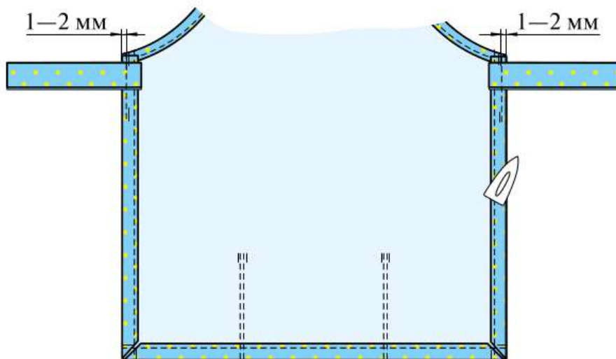
Рис. 6.44. Окончательная отделка фартука
