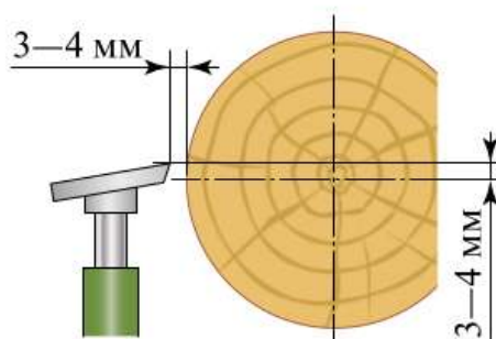
Рис. 4.31. Установка подручника
