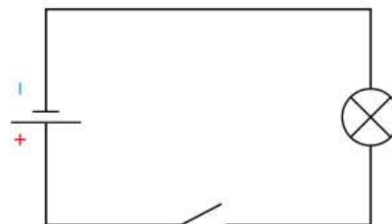
Рис. 11.15. Принципиальная схема однолампового осветителя
