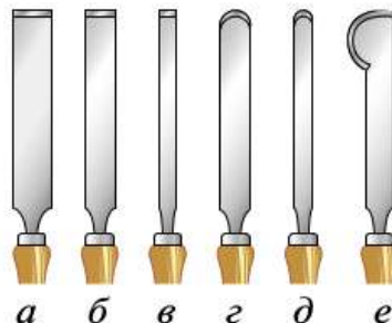
Рис. 4.24. Резцы-стамески:
