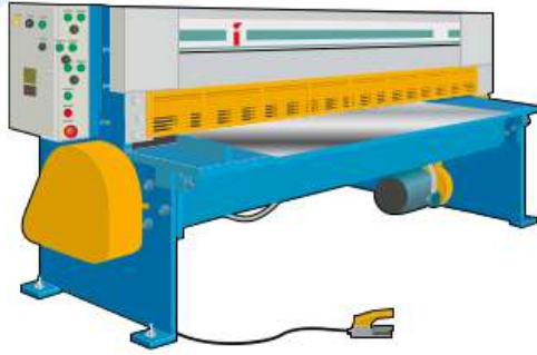
Рис. 5.23. Гильотинные ножницы
