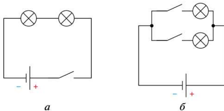
Рис. 11.12. Последовательное (а) и параллельное (б) включение ламп
