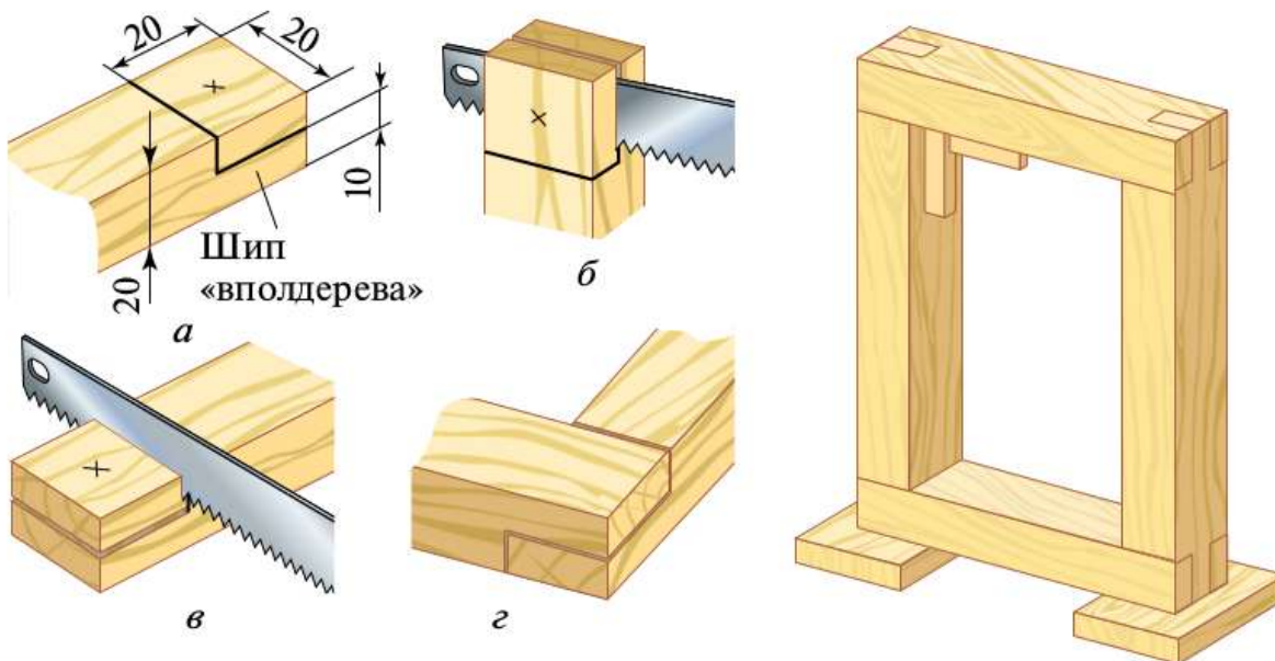
Рис. 4.58. Последовательность изготовления шипа «вполдерева»:
