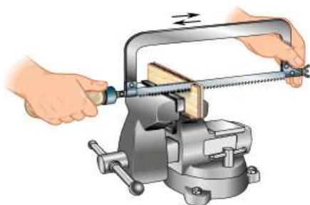
Рис. 5.27. Резание тонколистового металла
