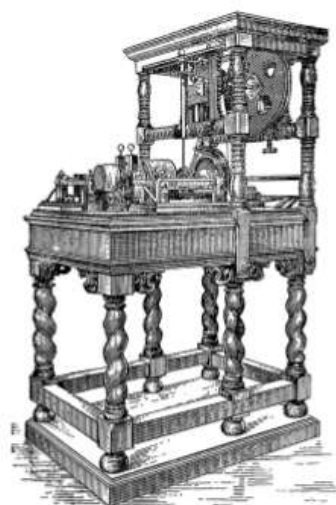
Рис. 4.4. Токарно-копировальный станок А. Нартова (1712)
