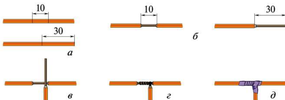
Рис. 11.5. Последовательность ответвления многожильных проводов
