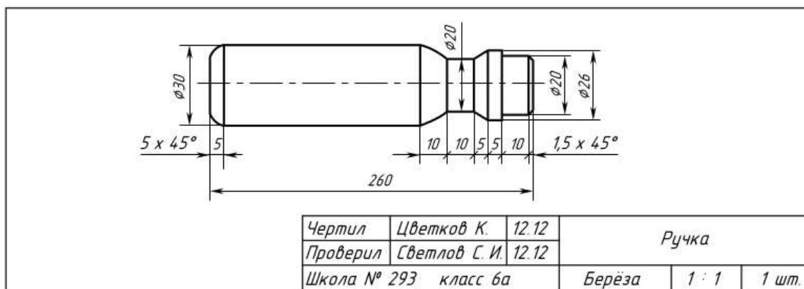
Рис. 4.40. Чертёж ручки резца-стамески
