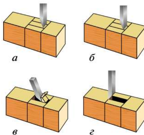
Рис. 4.56. Последовательность долбления гнезда
