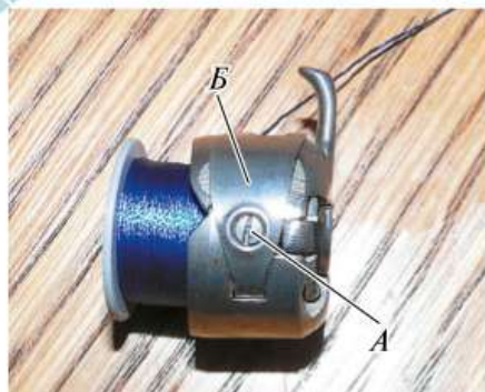
Рис. 6.14. Регулирование натяжения нити шпульного колпачка
