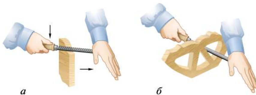
Рис. 4.46. Приёмы обработки: а — рашпилем; б — напильником
