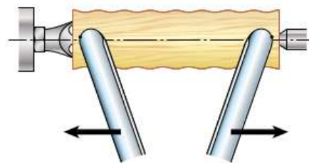
Рис. 4.33. Приёмы точения боковыми частями лезвия стамески
