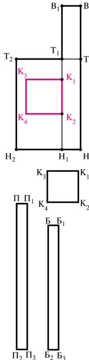
Рис. 6.22. Чертеж основы фартука с нагрудником
