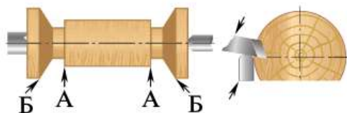
Рис. 4.37. Приёмы торцевания заготовки
