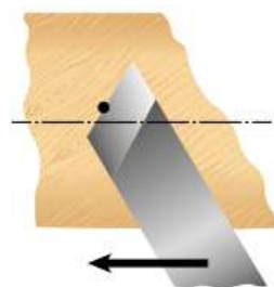
Рис. 4.34. Приём точения стамеской с косым срезом
