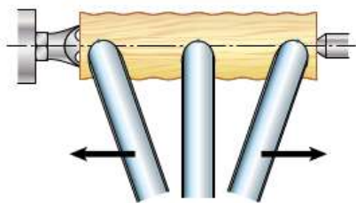
Рис. 4.32. Приёмы точения средней частью лезвия стамески
