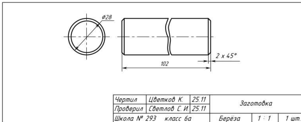
Рис. 4.39. Чертёж цилиндрической заготовки
