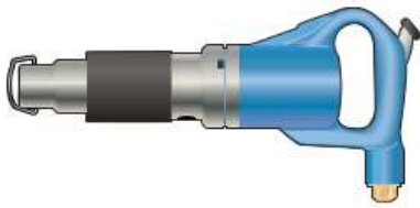
Рис. 5.51. Клепальный пневматический молоток
