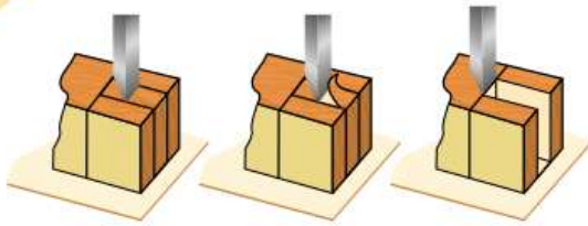
Рис. 4.57. Последовательность долбления сквозной проушины
