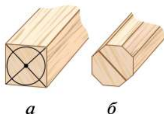
Рис. 4.25. Заготовка: а — разметка торцов; б — подготовленная заготовка
