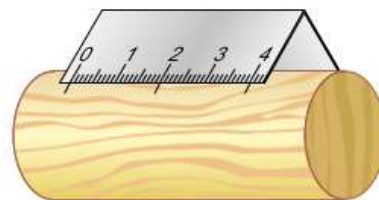
Рис. 4.19. Линейка с угловым подпором
