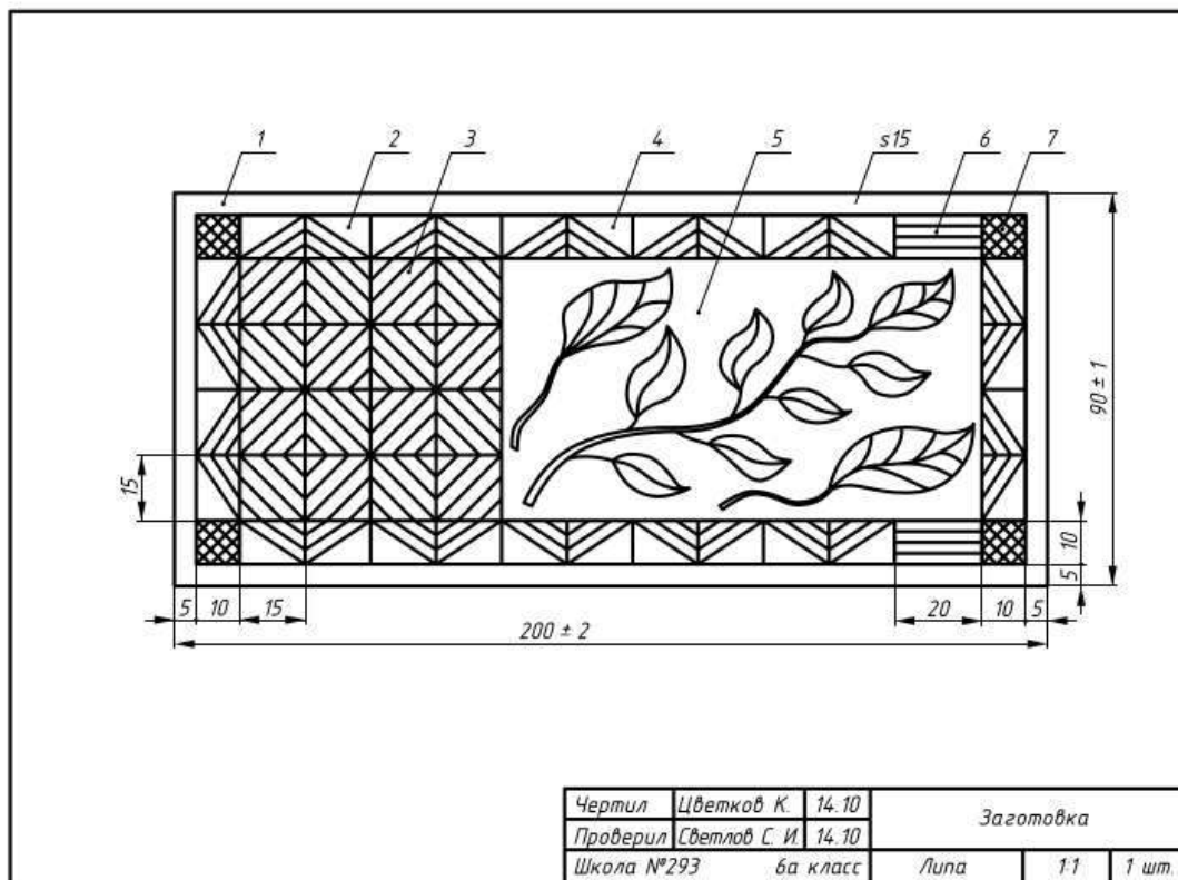
Рис. 8.7. Чертёж заготовки: 1 — контурное поле; 2 — орнаментальная полоса; 3 — резное поле из 16 квадратов 15 \times 15 мм; 4 — свободные места на орнаментальной полосе; 5 — резное поле; 6 — прямоугольник; 7 — квадрат 10 \times 10 мм
