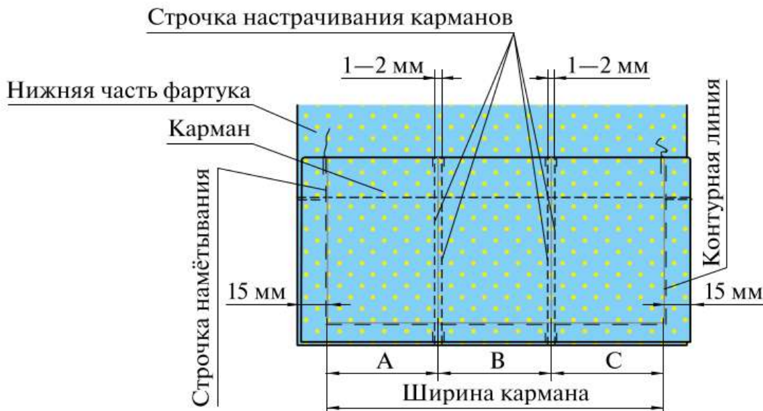
Рис. 6.41. Настрочивание кармана
