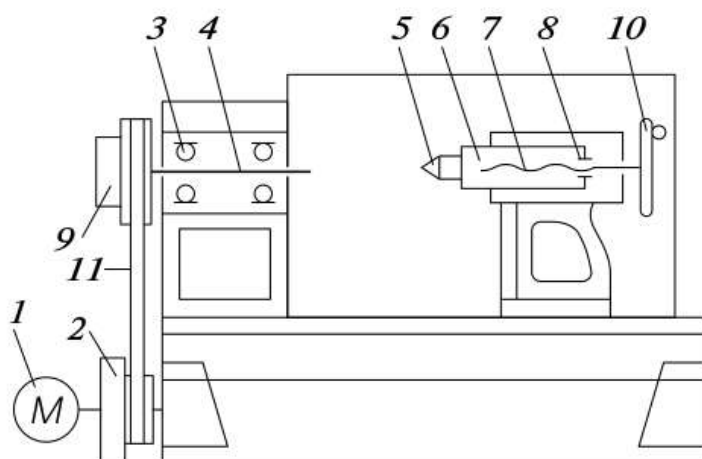
Рис. 3.6. Кинематическая схема токарного станка СТД-120М:
