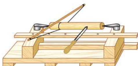
Рис. 4.3. Модель древнеегипетского станка с лучковым ручным приводом
