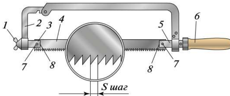
Рис. 5.24. Ручная слесарная ножовка с раздвижной рамкой
