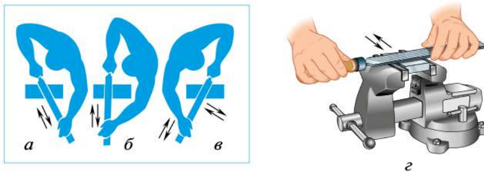
Рис. 5.36. Приёмы опиливания: а — косым штрихом; б — поперечным штрихом; в — перекрёстным штрихом; г — продольным штрихом
