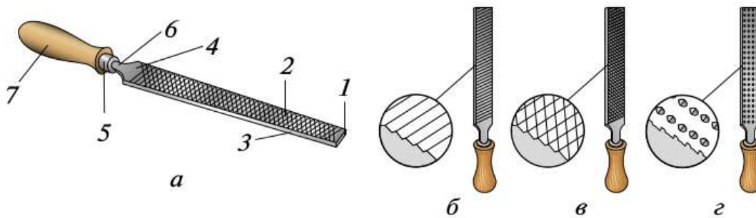
Рис. 5.31. Напильники: а — основные части: 1 — нос; 2 — ребро; 3 — грань; 4 — пятка; 5 — кольцо; 6 — хвостовик; 7 — ручка; б — одинарная (простая) насечка; в — двойная (перекрёстная) насечка; г — рашпильная насечка
