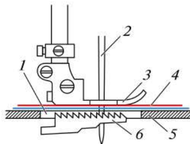
Рис. 6.16. Взаимодействие прижимной лапки и зубчатой рейки:
