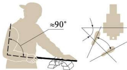
Рис. 5.34. Рабочее положение при опиливании
