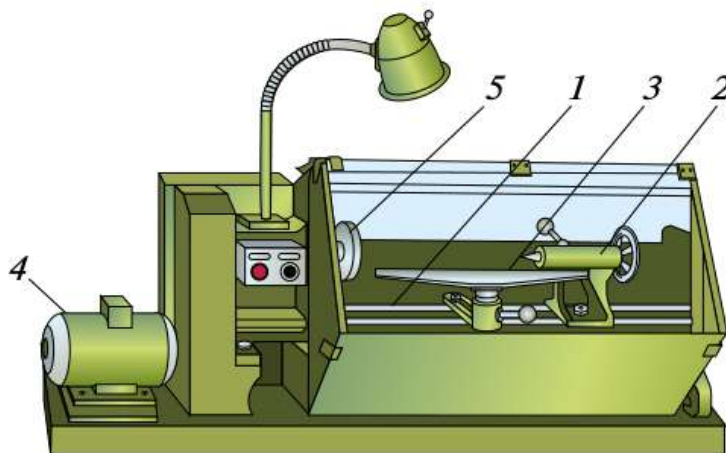
Рис. 4.9. Токарный станок для обработки древесины
