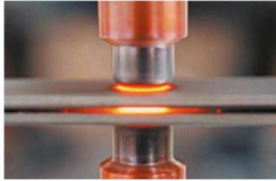
Рис. 2.10. Процесс контактной электросварки
