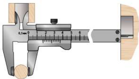
Рис. 4.14. Приёмы измерения древесины штангенциркулем
