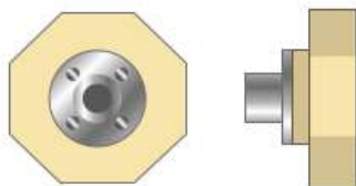
Рис. 4.28. Крепление заготовки к планшайбе
