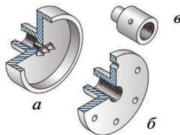
Рис. 4.26. Крепёжные приспособления: а — резубец; б — планшайба; в — патрон-стакан
